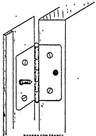
BISAGRA CON TRANCIL
